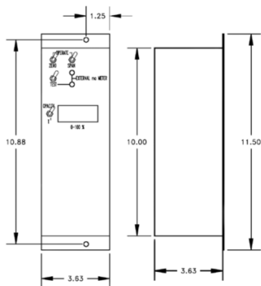
OPM 4001 Service Module
